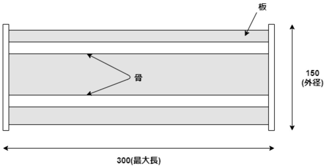
上面図
